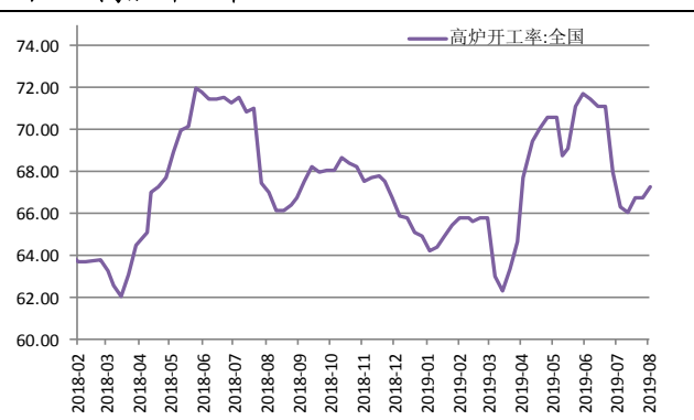
图 9：高炉开工率
