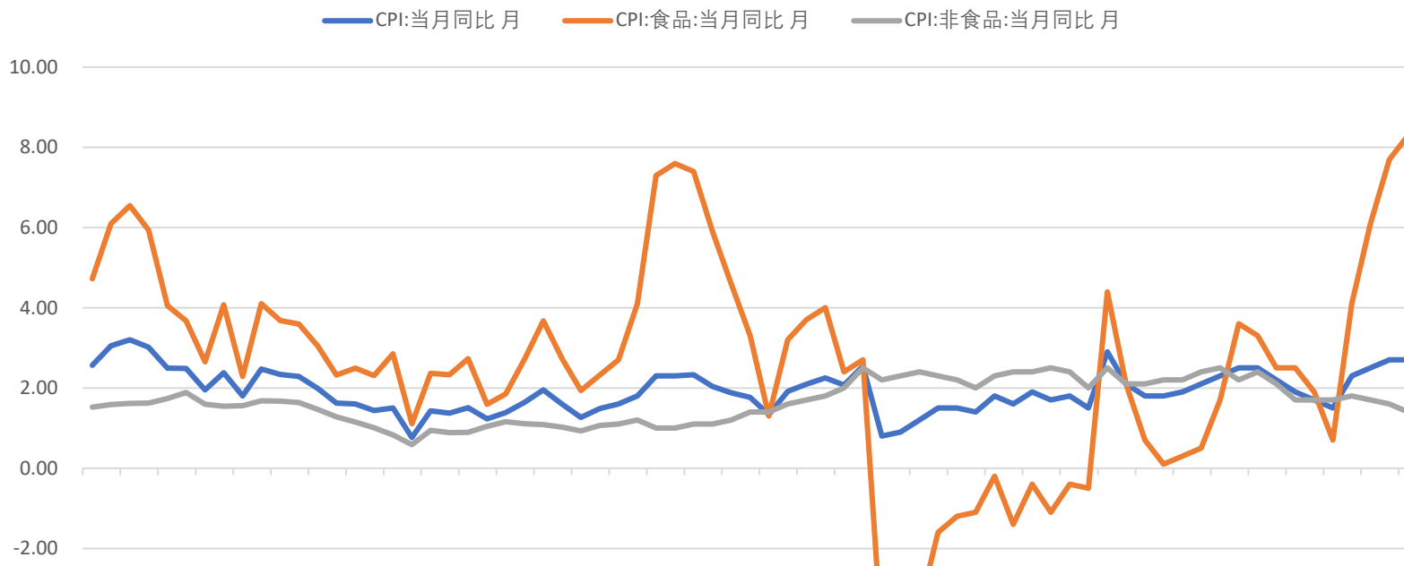
图：6月CPI
