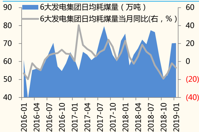
图表 3：6 大发电集团日均煤耗同比跌幅扩大
