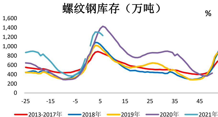
图 6：螺纹钢库存
