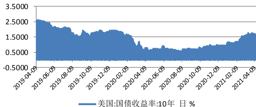
图 2 (十年期美债收益率, %)
