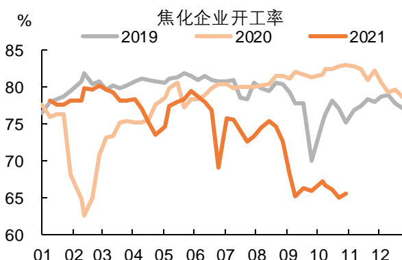
图表6 本周焦化企业开工率65.5%，处于年内低点
