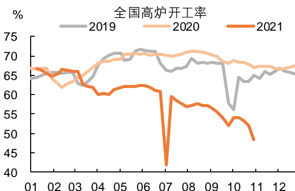
图表4 本周全国高炉开工率48.5%，降至年内次低
