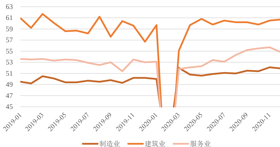
图 3 制造业、服务业以及建筑业 PMI 指数比较（单位：%）
