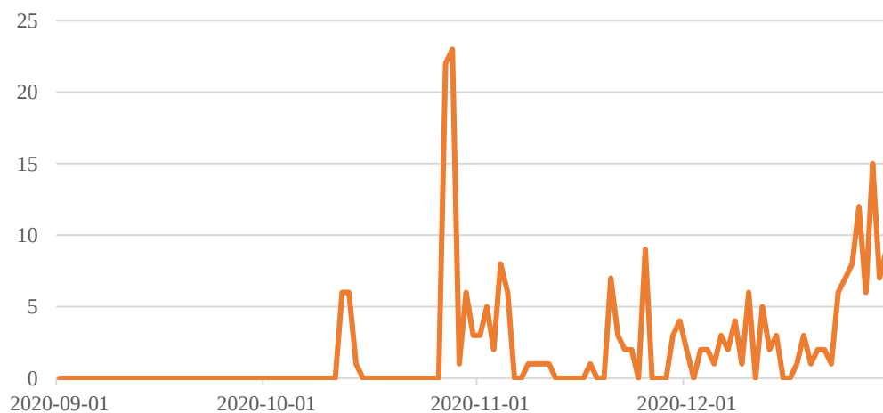
图 4 9 月以来全国当日新增本土确诊病例（单位：例）
