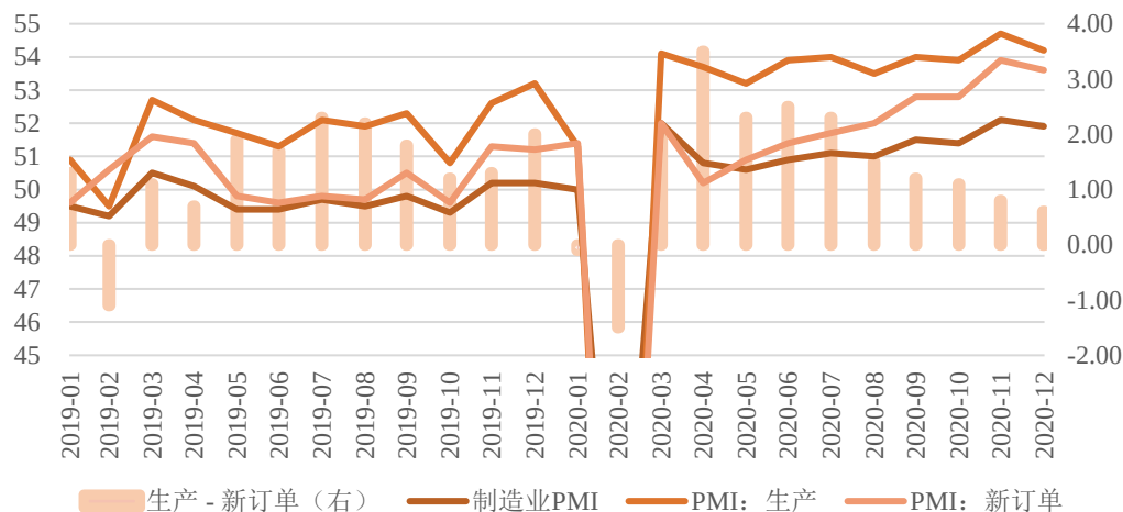
图1 制造业PMI及其分项指标比较（单位：%）
