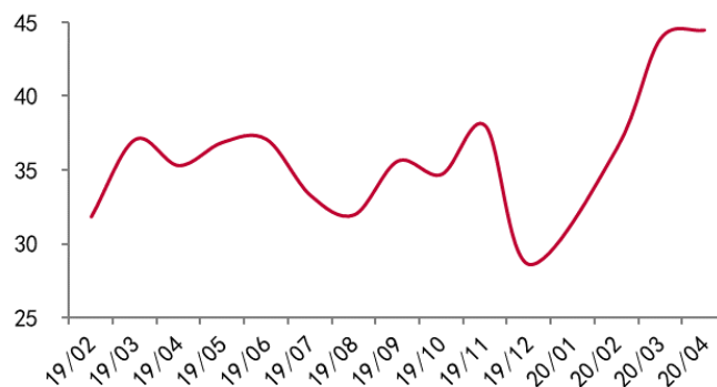
图表 7: 农村居民用电量占比 (%)
