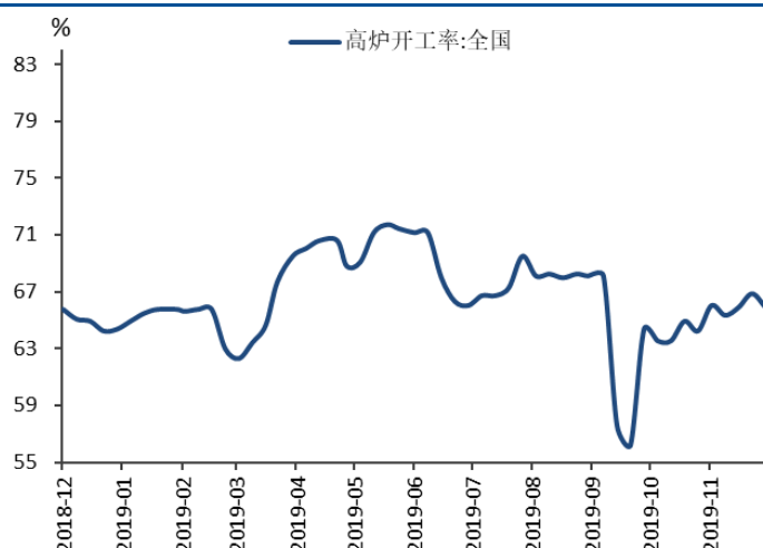
图 7：高炉开工率 (%)
