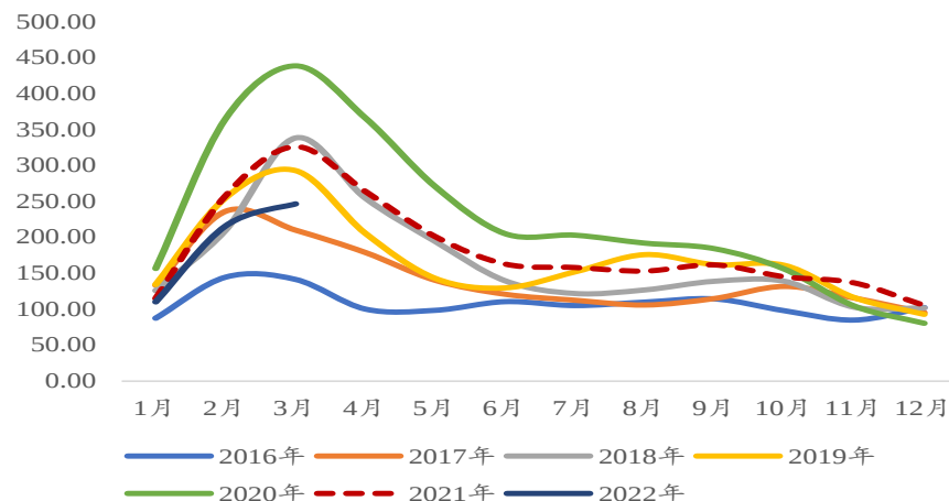
线材库存（万吨）
