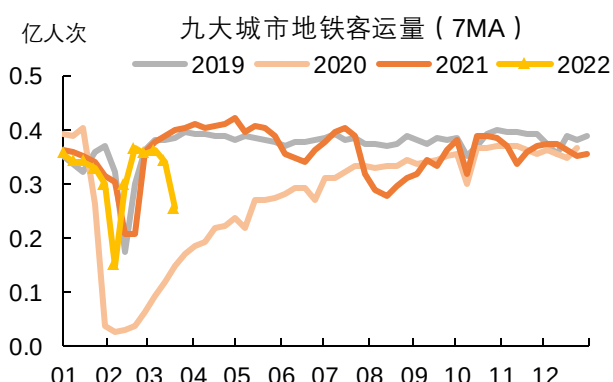
图表20 本周 9 大城市日均地铁客运量 2529 万,环比下滑 25.5%
