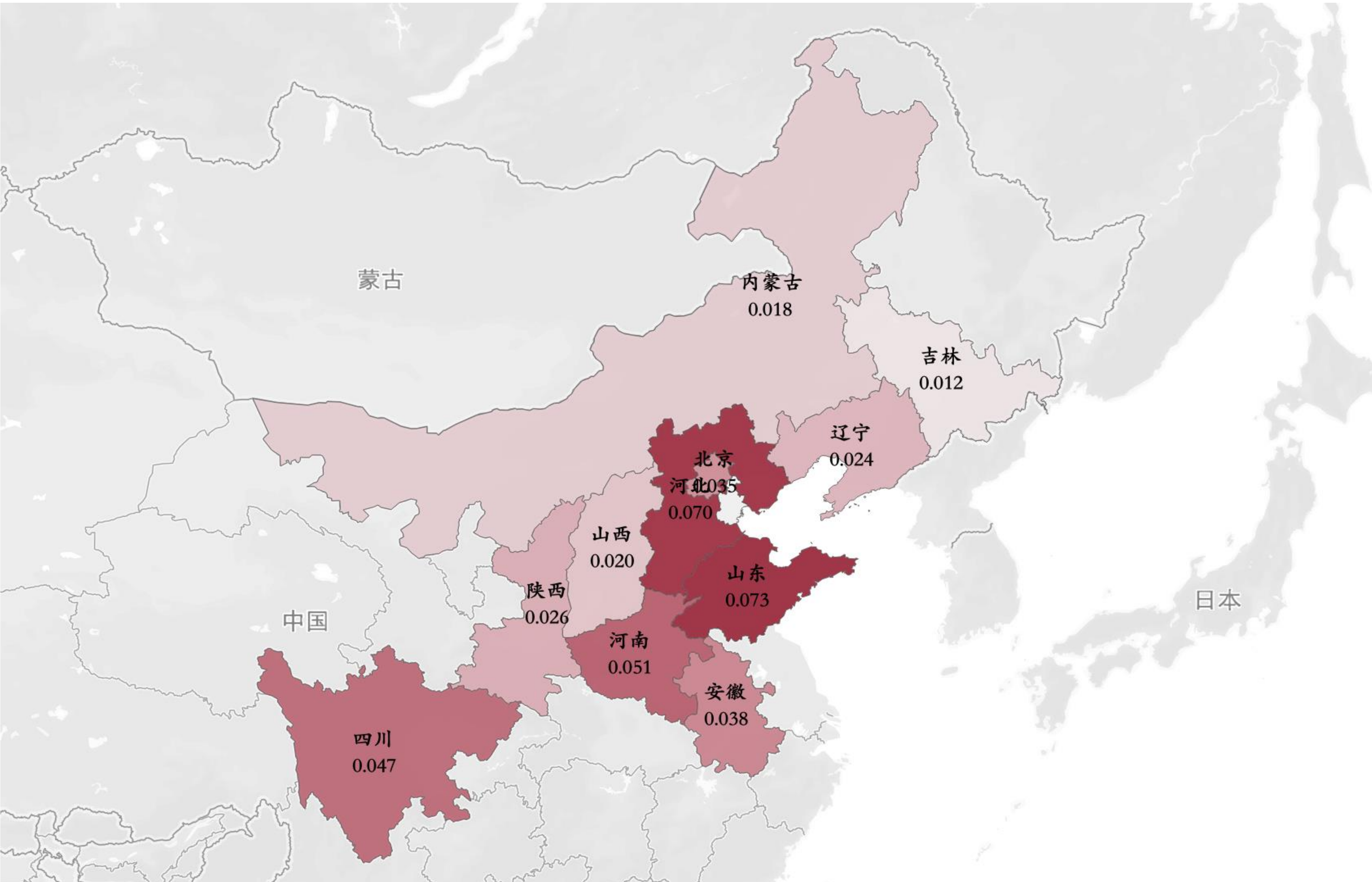
图二 受冷空气影响严重省份/市的GDP占比
