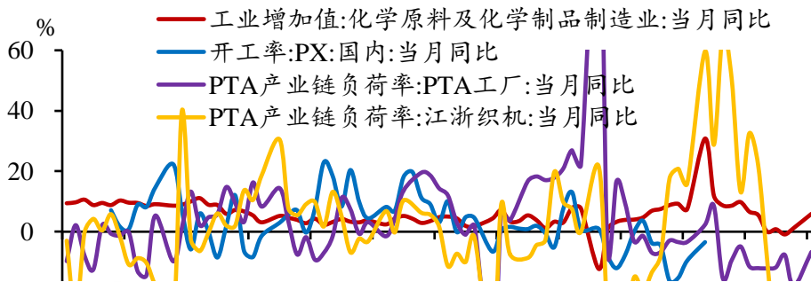
图 5：化工行业高频指标同比与化学原料及制品增加值同比
