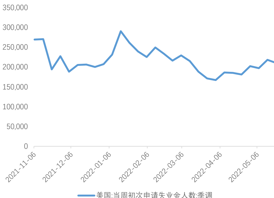
图 3: 首申人数激增至 21.8 万人
