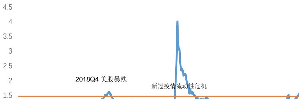
图 5：投资级债券利差回升至关键点位（%）
