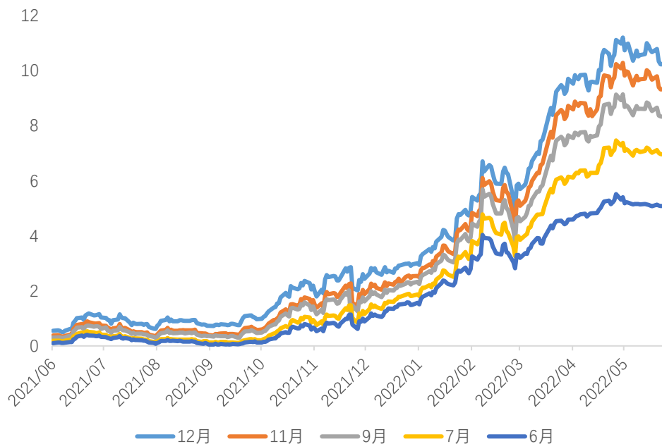
图 1：6/7/9/11/12 月隐含加息次数
