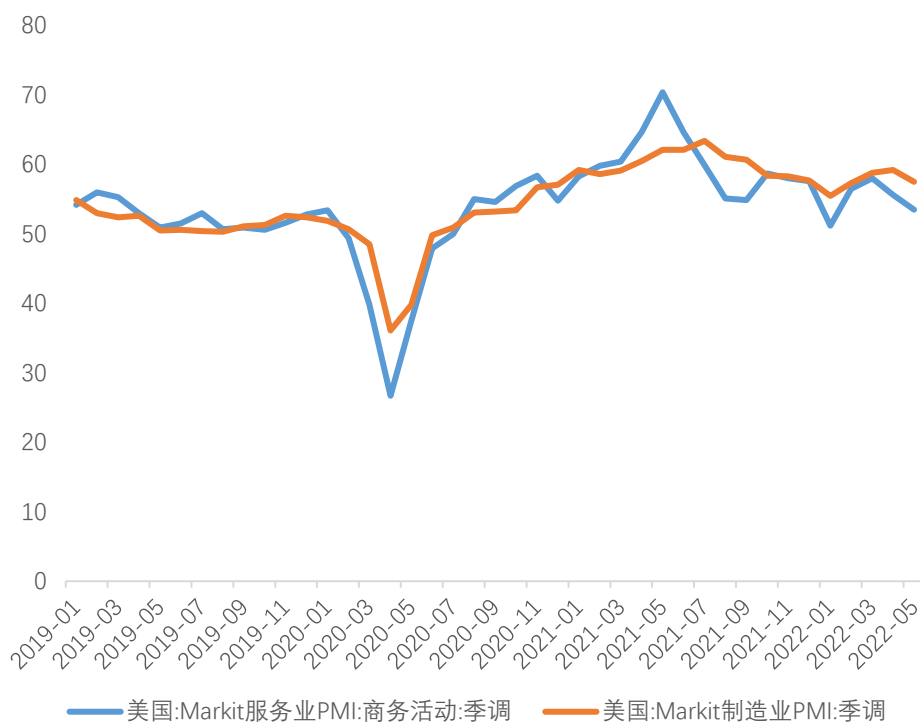
图 2: Markit5 月数据出现回落
