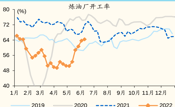
图表 8: 炼油厂开工率较上周提升
