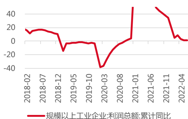
图1 (工业企业利润累计同比增速, %)
