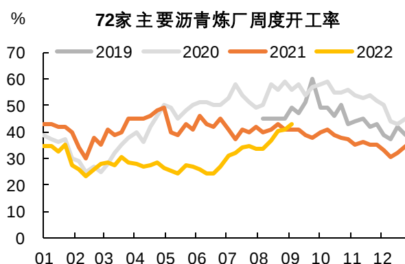
图表8 72 家主要沥青炼厂开工率环比上升 2.1 个百分点
