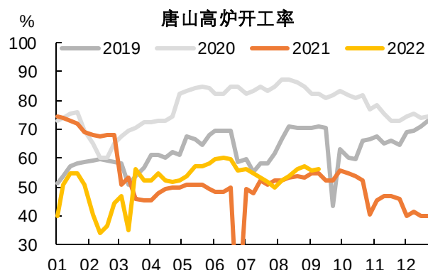
图表6 本周唐山高炉开工率环比提升 0.8 个百分点
