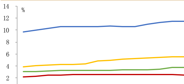
图 4：粤港澳、长三角、成渝城市群常住人口占全国比重提升
