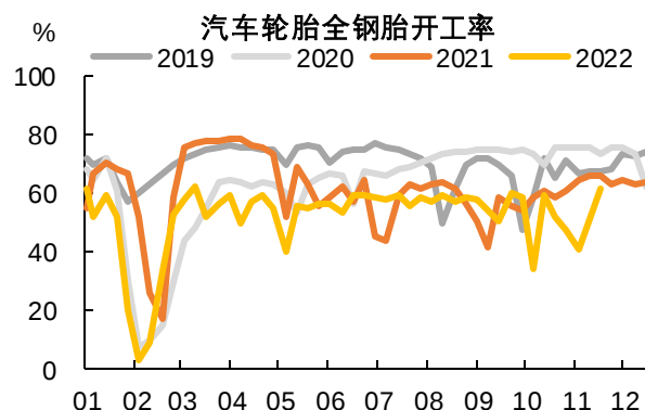
图表11 本周汽车轮胎全钢胎开工率 61.6%，环比上升 10.6 个百分点
