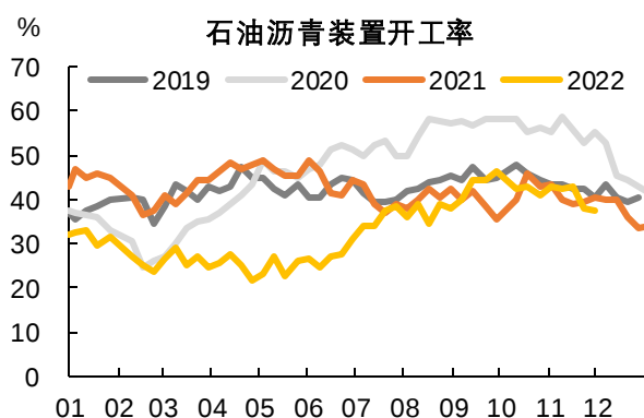
图表8 本周石油沥青装置开工率 37.6%，环比降 0.6 个百分点
