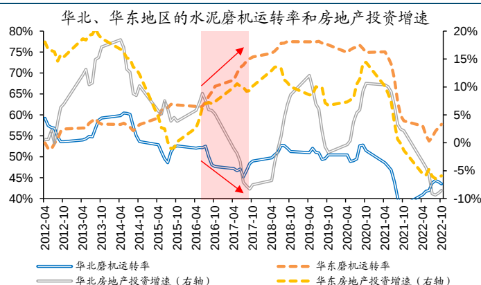
图表8：华北华东水泥生产分化映射两地地产投资分化
