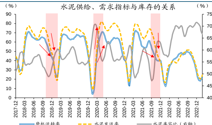
图表12：水泥供需相对变化可通过库存指标体现
