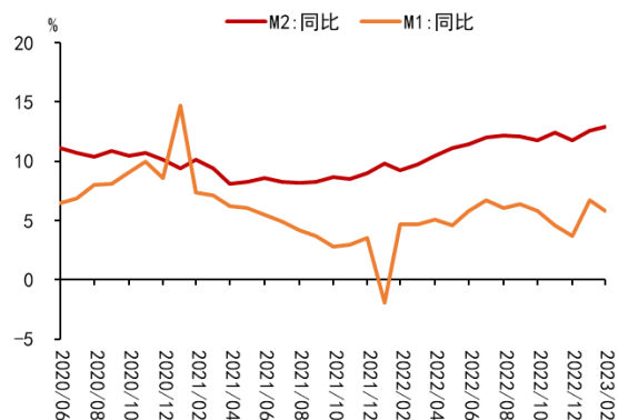
图 4：M1、M2 同比
