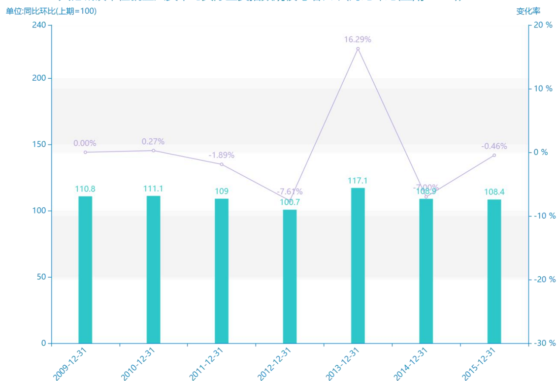
2009-2015其他城镇单位就业人员平均实际工资指数规模与增长率(同比环比(上期=100))
