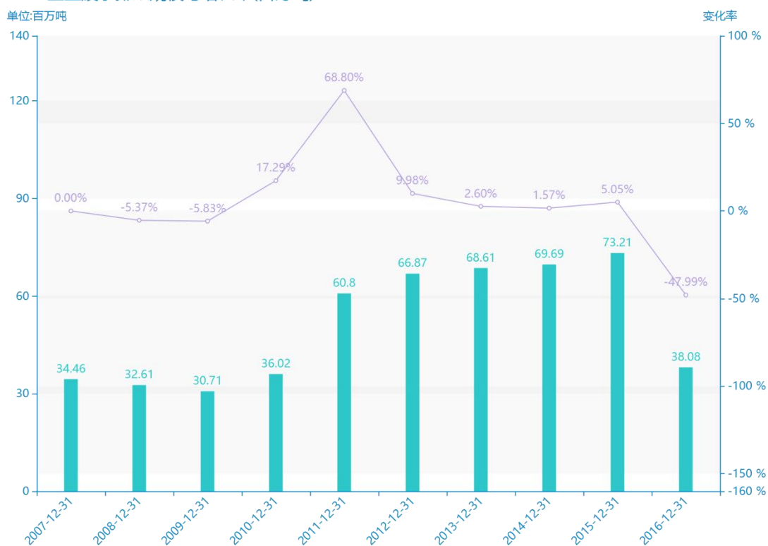
2007-2016工业废水排放规模与增长率(百万吨)
