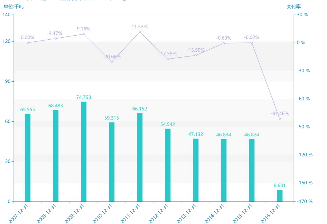
2007-2016二氧化硫排放量规模与增长率(千吨)
