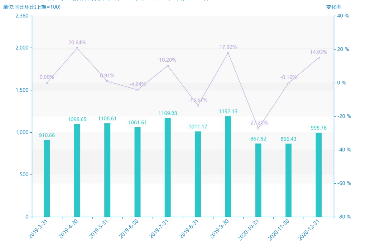
2019-2020义乌鞋景气指数规模与增长率(同比环比(上期=100))
