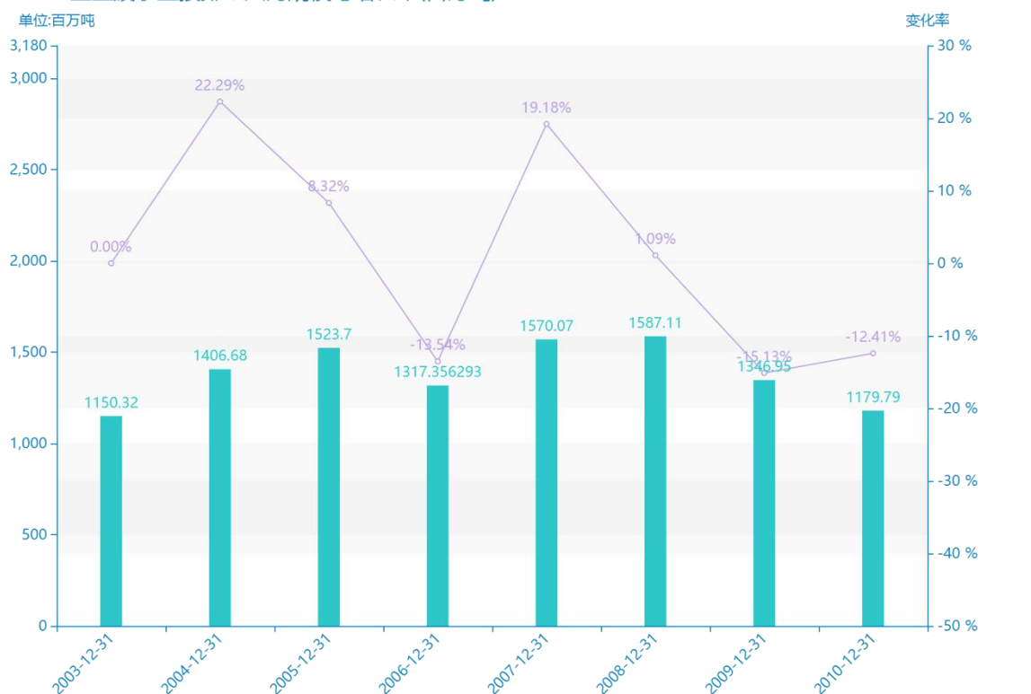
2003-2010工业废水直接排放入海规模与增长率(百万吨)
