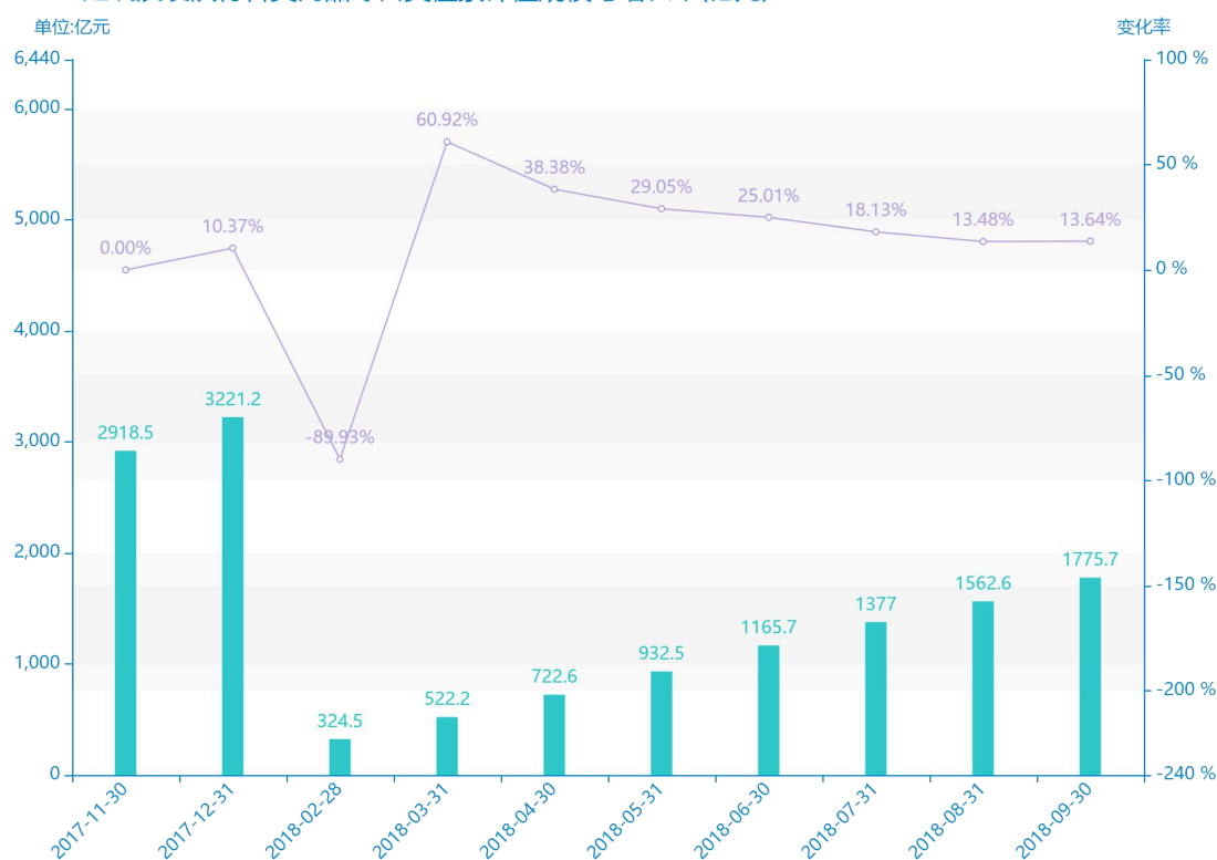
2017-2018建筑及装潢材料类商品零售类值累计值规模与增长率(亿元) ■ 建筑及装潢材料类商品零售类值累计值(亿元) —○— 增长率
