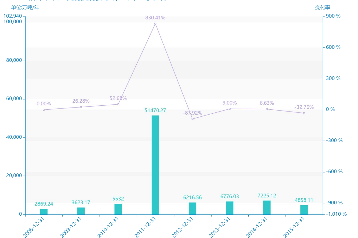
2008-2015铅锌采矿建设规模与增长率(万吨每年)
