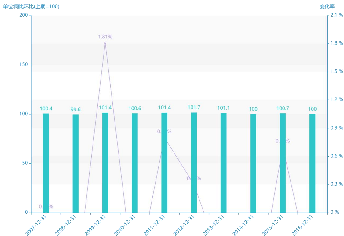
2007-2016 文化娱乐类居民消费价格指数规模与增长率(同比环比(上期=100)) 文化娱乐类居民消费价格指数(上年=100) —○— 增长率
