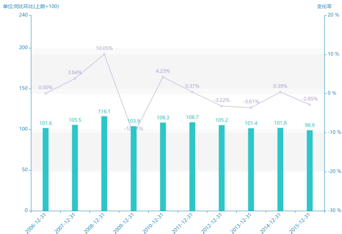
2006-2015水产品类商品零售价格指数规模与增长率(同比环比(上期=100)) 水产品类商品零售价格指数(上年=100) —○— 增长率
