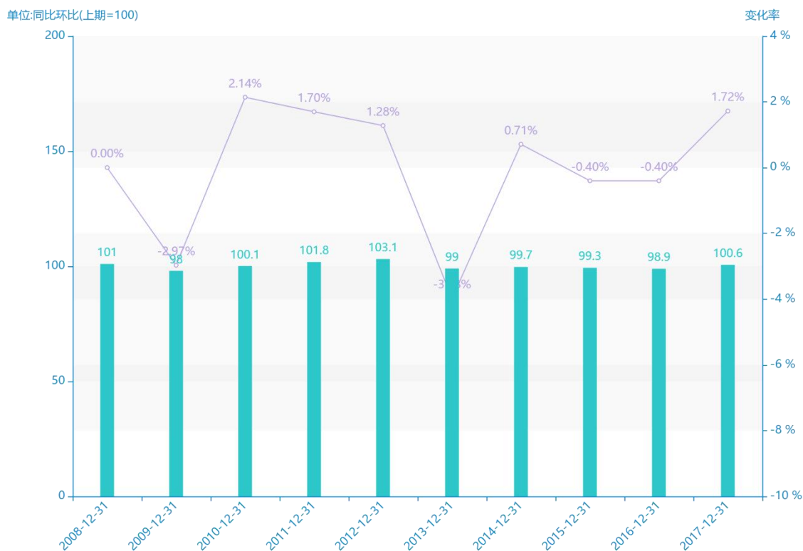
2008-2017设备工器具购置固定资产投资价格指数规模与增长率(同比环比,上期=100)
