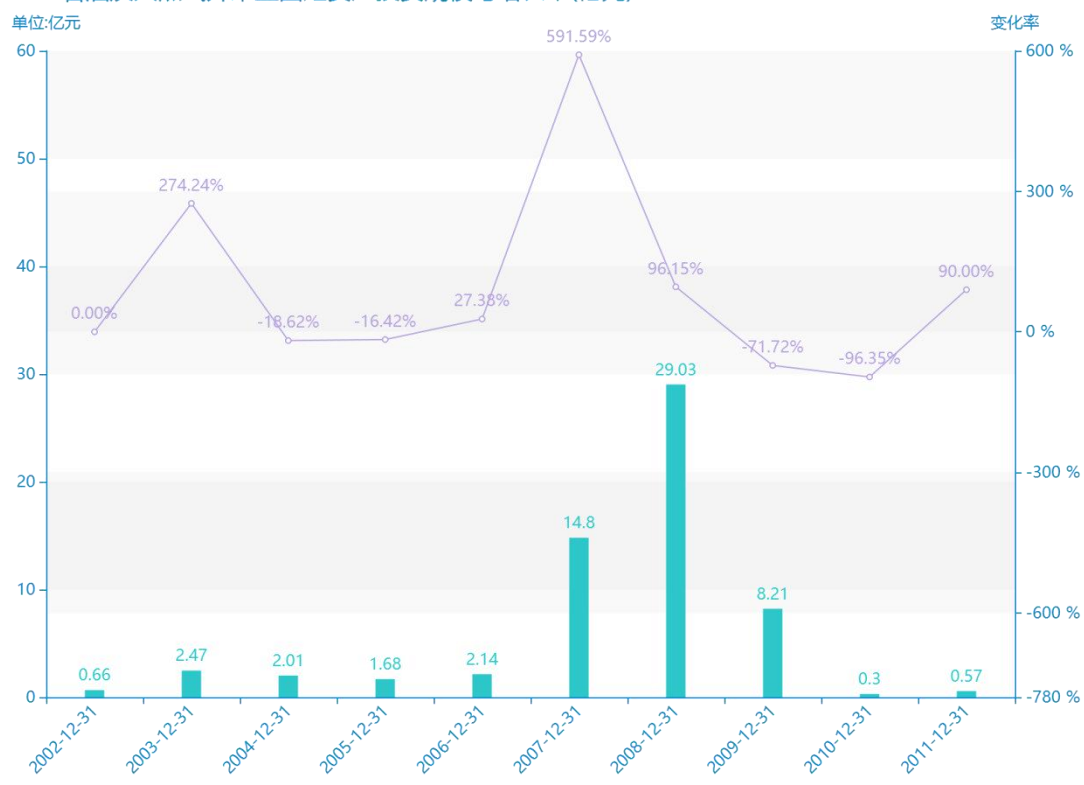
2002-2011石油及天然气开采业固定资产投资规模与增长率(亿元) 石油及天然气开采业固定资产投资(不含农户)(亿元) —○— 增长率
