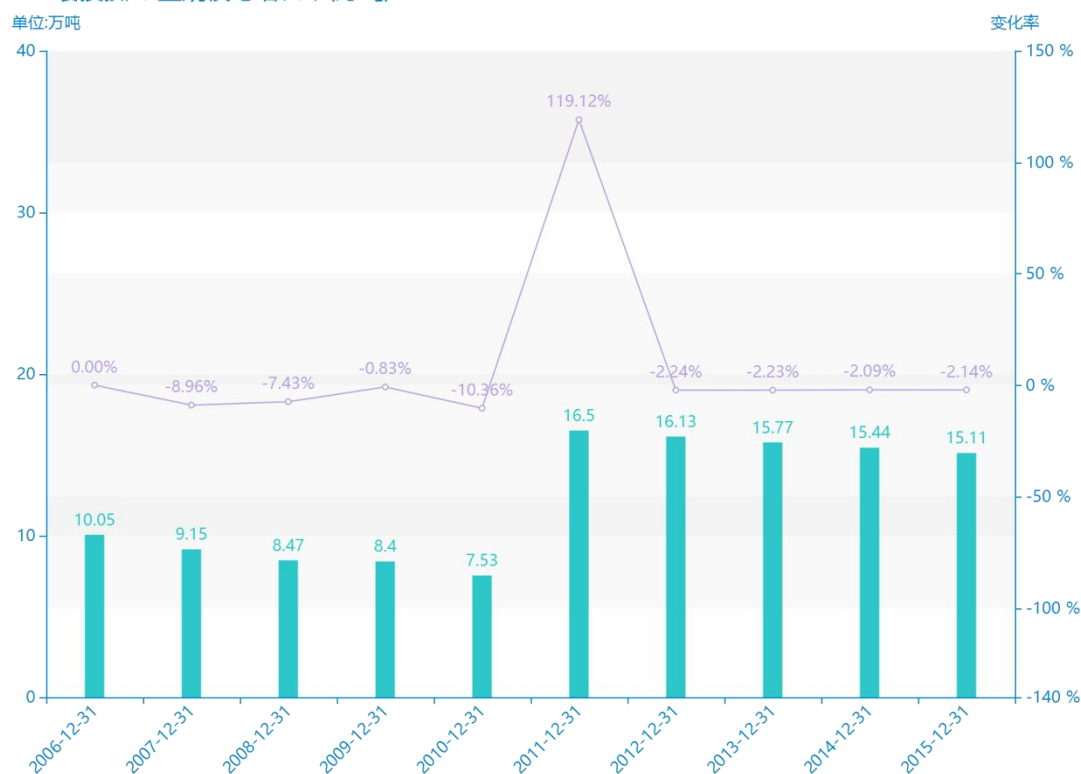
2006-2015氨氮排放量规模与增长率(万吨)
