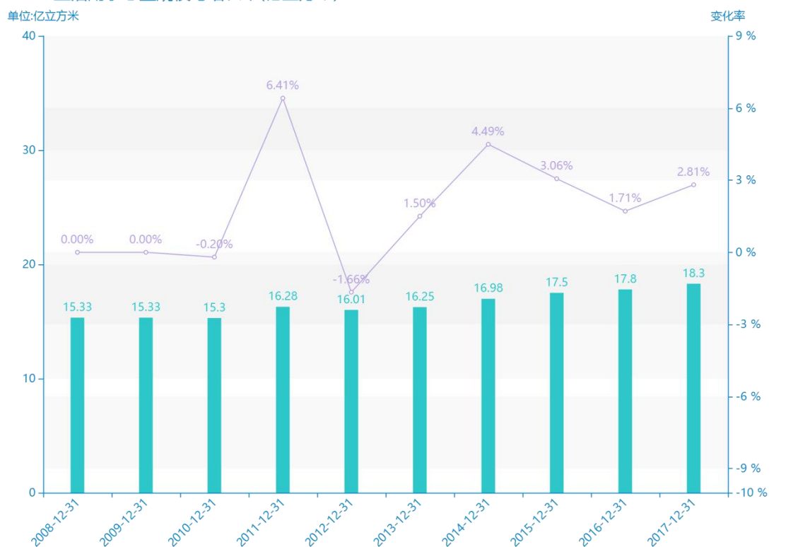
2008-2017生活用水总量规模与增长率(亿立方米)
