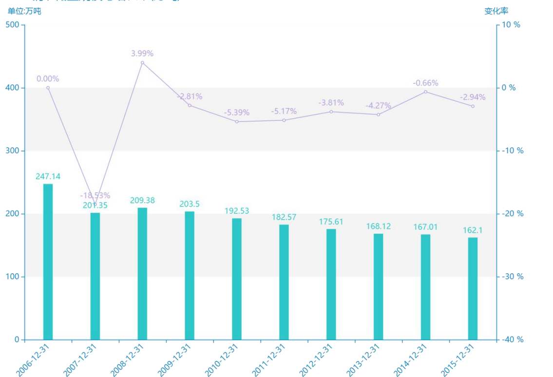
2006-2015铜矿储量规模与增长率(万吨)
