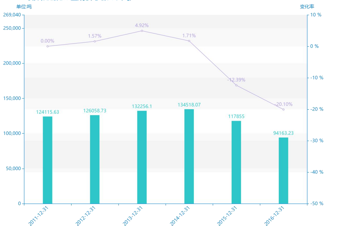
2011-2016氮氧化物排放量规模与增长率(吨)
