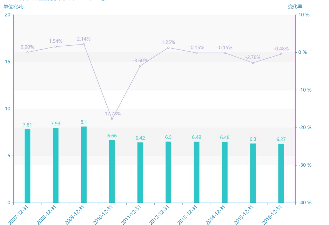
2007-2016磷矿储量规模与增长率(亿吨)
