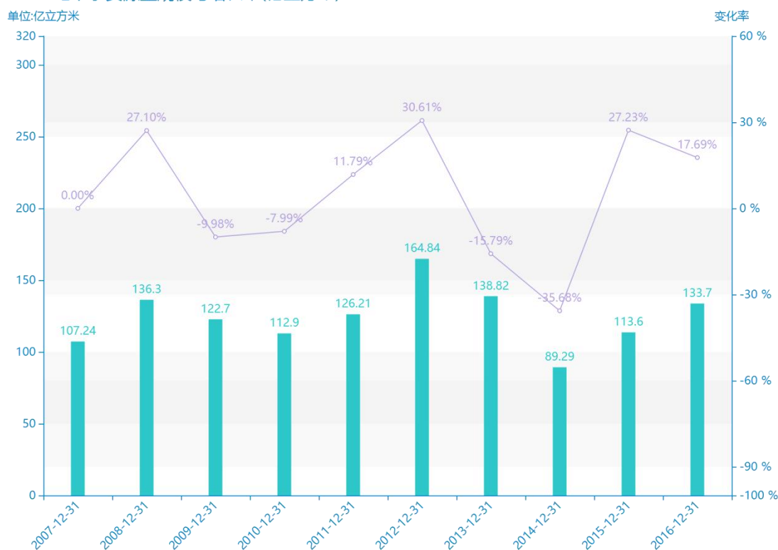
2007-2016地下水资源量规模与增长率(亿立方米)
