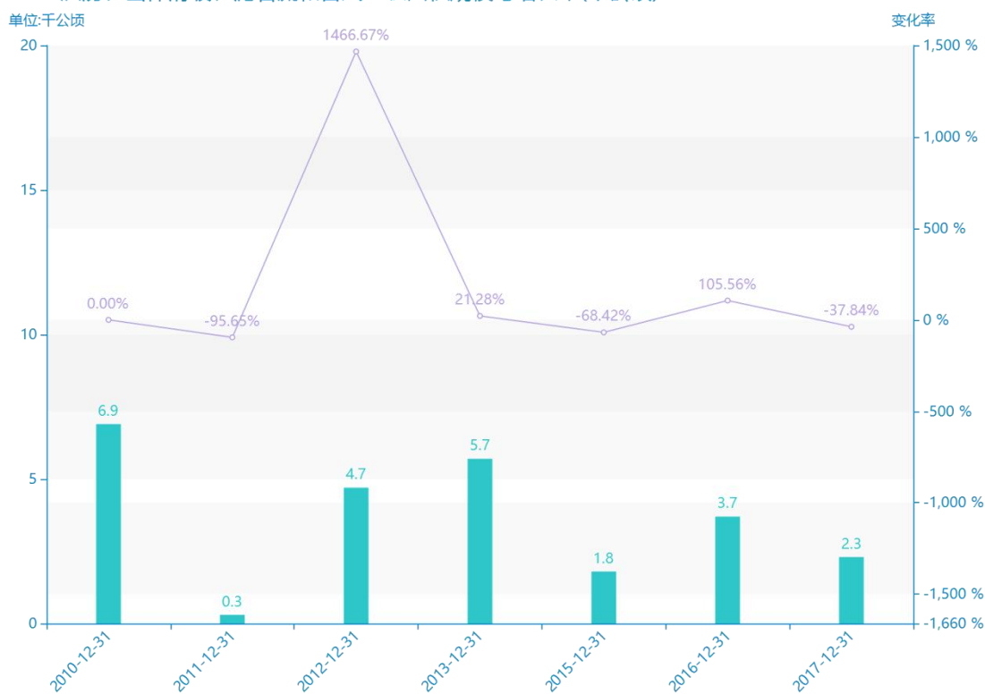
2010-2017洪涝、山体滑坡、泥石流和台风绝收面积规模与增长率(千公顷) —○— 增长率
