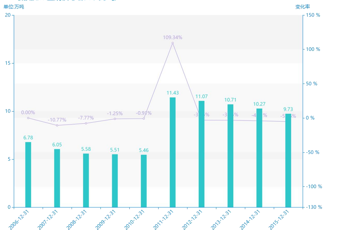
2006-2015氨氮排放量规模与增长率(万吨)
