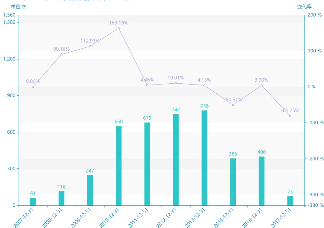
2007-2017发生地质灾害起数规模与增长率(次)
