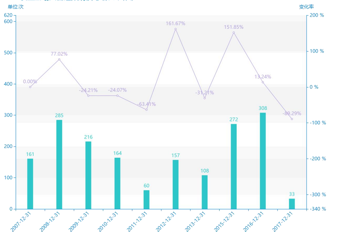
2007-2017发生崩塌灾害起数规模与增长率(次)
