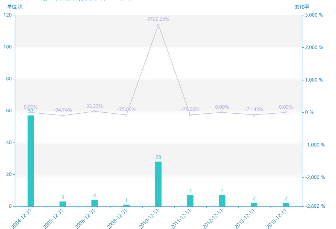
2004-2015发生崩塌灾害起数规模与增长率(次)
