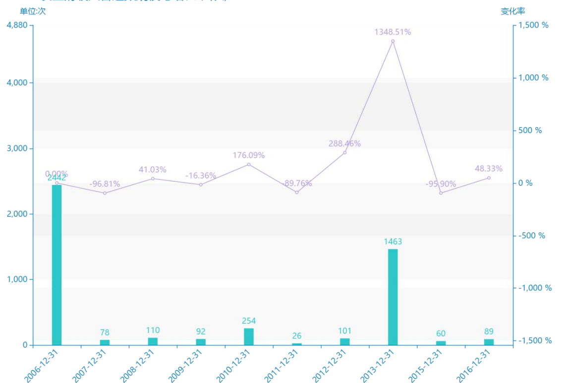
2006-2016发生滑坡灾害起数规模与增长率(次)
