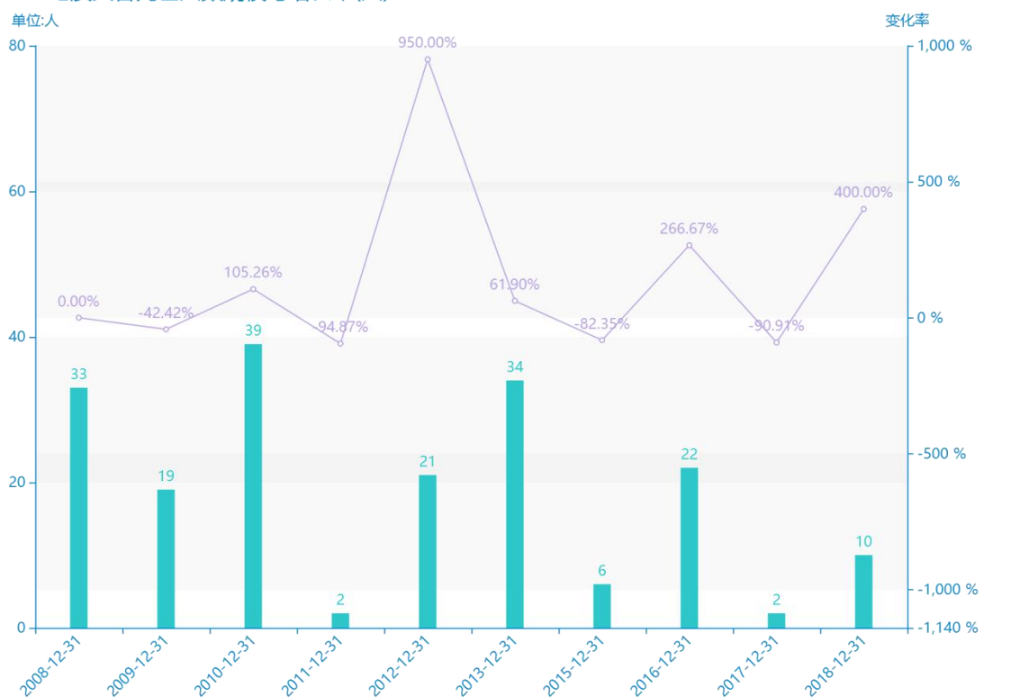
2008-2018地质灾害死亡人数规模与增长率(人)
