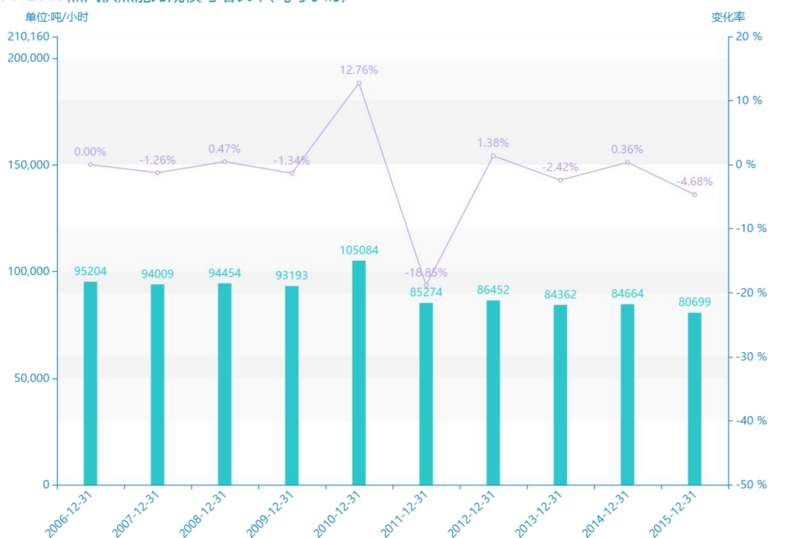
2006-2015蒸汽供热能力规模与增长率(吨每小时)
