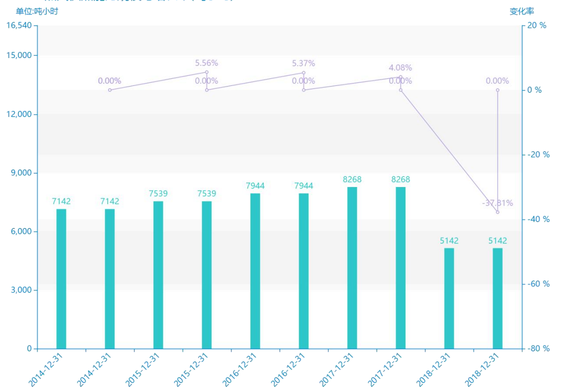
2014-2018蒸汽供热能力规模与增长率(吨小时)
