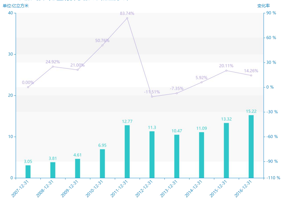
2007-2016天然气供气总量规模与增长率(亿立方米)
