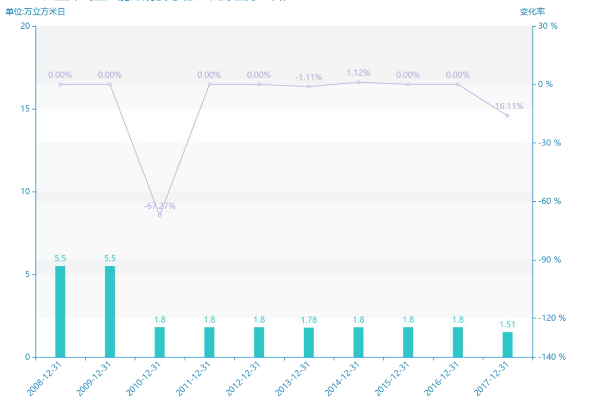
2008-2017人工煤气生产能力规模与增长率(万立方米日)
